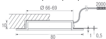
Установка светильника
