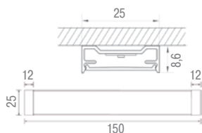
Установка светильника
