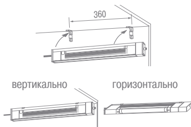
Варианты установки:
