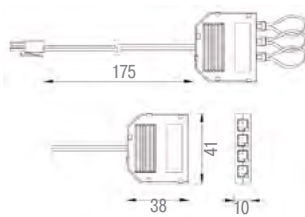
Габаритные размеры
