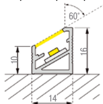
Габаритные размеры
