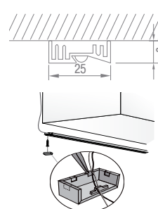
Установка светильника:
