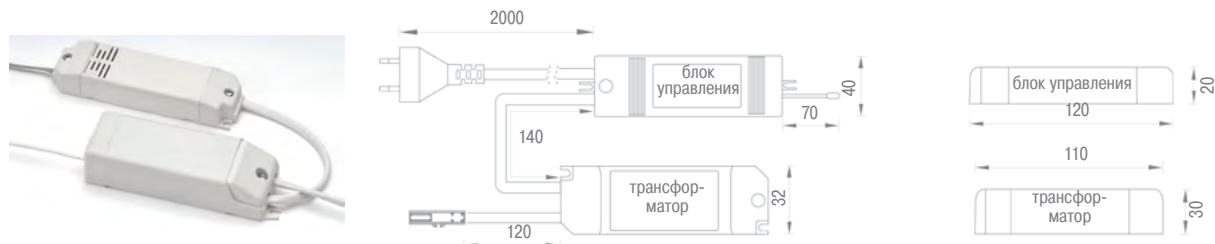
Подключение светильника ODO CUCINA к трансформатору с включением от касания
