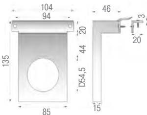
Установка светильника
