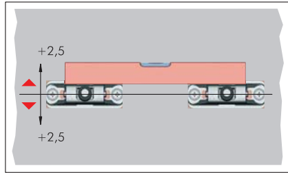
2. Отрегулировать крепления.
