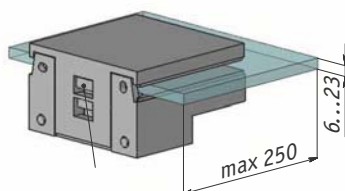
Положение скобы для плиты от 6 мм до 23 мм
