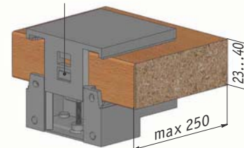
Положение скобы для плиты от 23 мм до 40 мм
