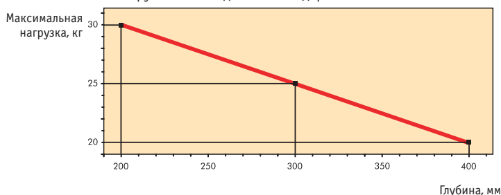
Соотношение между глубиной полки и нагрузкой на каждый менсолдержатель
