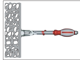
3. Затянуть фиксирующие саморезы.
