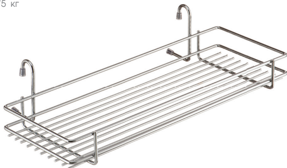
Полка широкая 450x215x105 мм 0,75 кг
